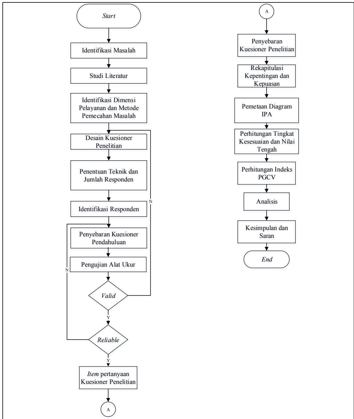
Gambar 3.1 Metodologi Penelitian
