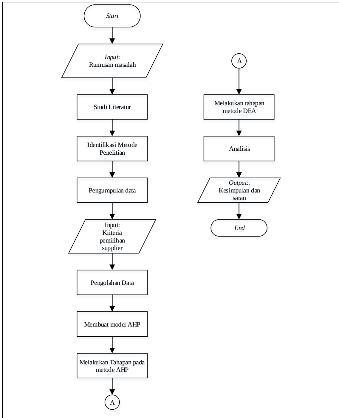
Gambar 3. 1 Metodologi Penelitian
